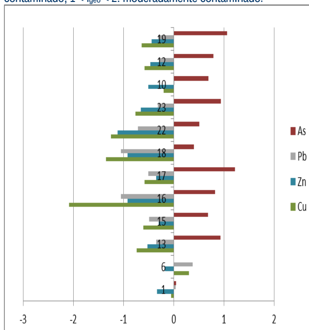
Imagen 3. I_{geo} calculados para las muestras de sedimentos de la presa. Zn: zinc, Cu: cobre, Pb: plomo y As: arsénico. I_{geo} < 0: no contaminado; 0 < I_{geo} < 1: no contaminado a moderadamente contaminado; 1 < I_{geo} < 2: moderadamente contaminado.
